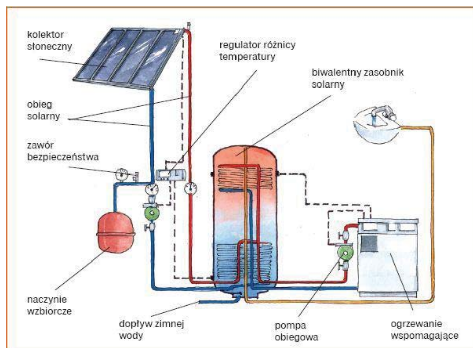
Ryc. 9. Schemat instalacji solarnej
